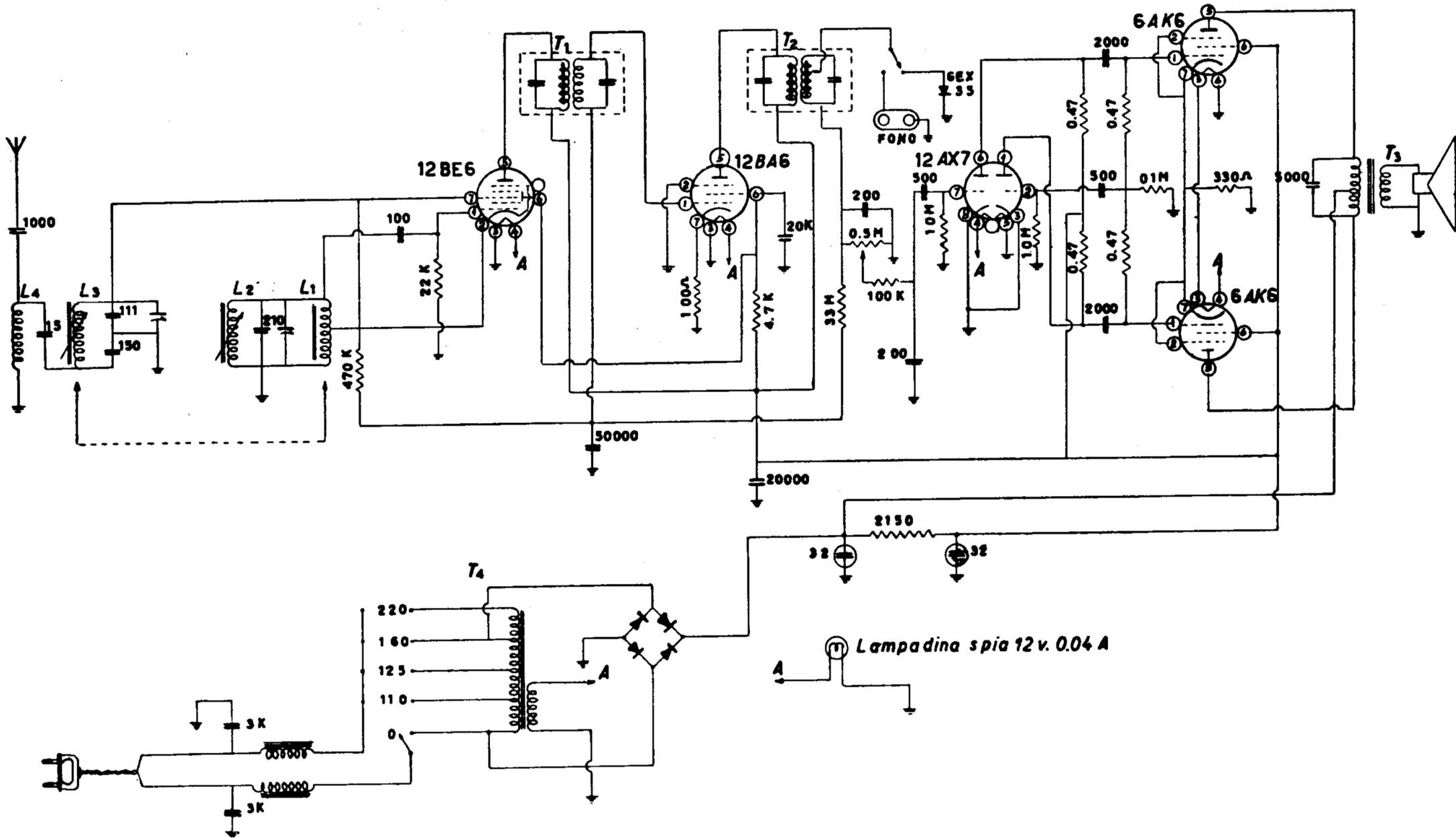
SICART-EMERSON - Mod. A 802. Gamma di ricezione: onde medie. Media frequenza 455 kc/s. Potenza di uscita 3 watt. Consumo 30 watt. Piccolo ricevitore di elevata potenza e qualità di riproduzione. Provvisto di circuito a bassa frequenza ad inversione di fase elettronica e di amplificazione in controfase finale.
